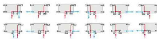
Rozšiřující možnosti připojení těles RADIK VKM8 na otopnou soustavu
