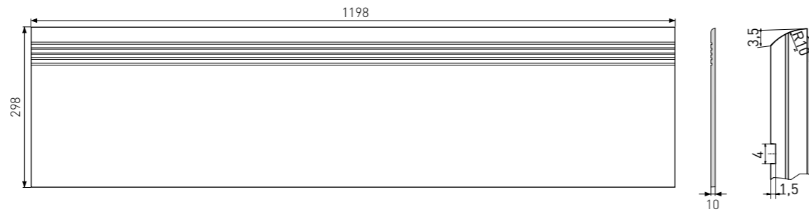
Stufe | DCPVF... | 298×1198×10 mm step tile | DCPVF... | 298×1198×10 mm
