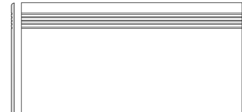
DCPSE735 běžová | beige DCPSE736 hnědá | brown DCPSE737 šedá | grey DCPSE738 tmavě šedá | dark grey DCPSE739 černá | black PEI 4-5 \varnothing 72 | ks mat | matt | R9 | A
