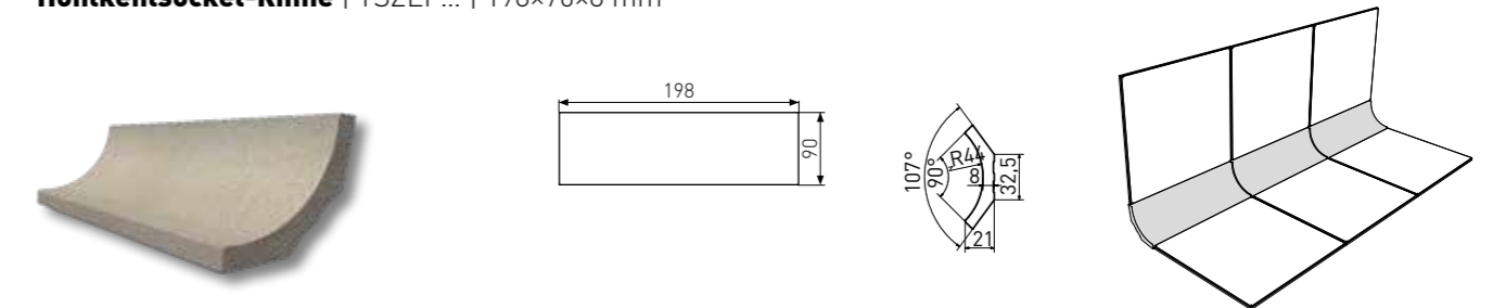
Hohlkehlsocle-Rinne | TSZEF... | 198×70×8 mm
