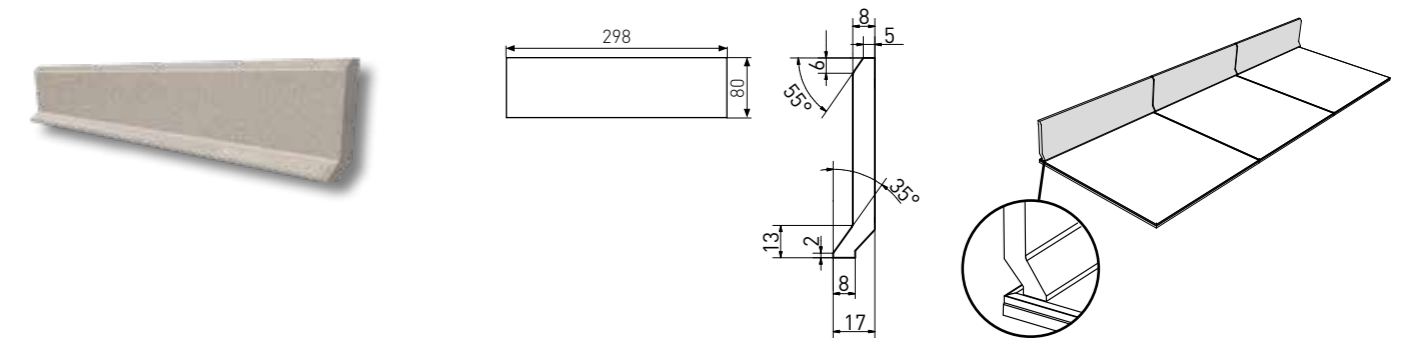
Französischer Sockel | TSFJB... | 298×80×9 mm
