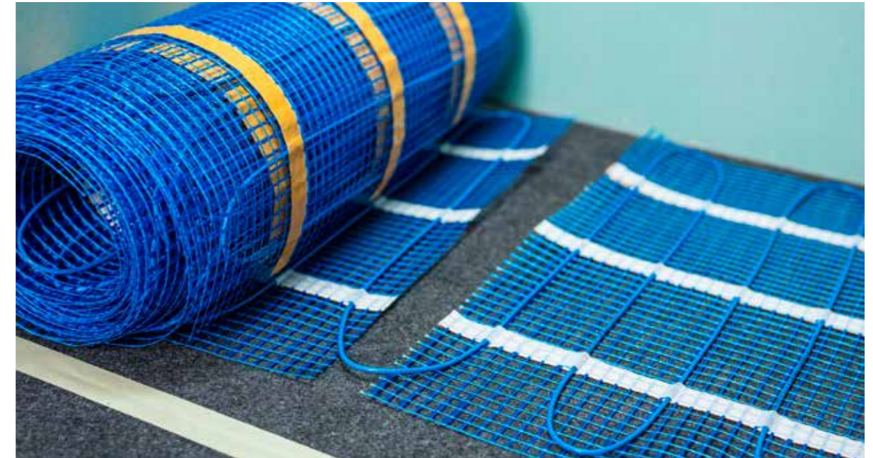
Bild 15 Elektrischer Raster mit Heizkabeln und dem DSDI-Paneel als Wärmeisolation
