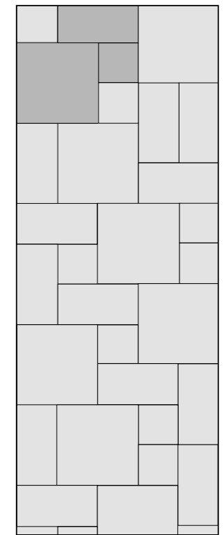
45 x 45 = 57 %, 22,5 x 45 = 29 %, 22,5 x 22,5 = 14 %
